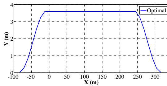
Fig11. The optimal trajectory for the same auto.
